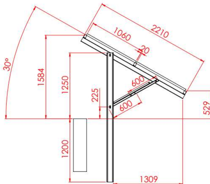
Слика 14. Приказ на монтажната конструкција со панелите
