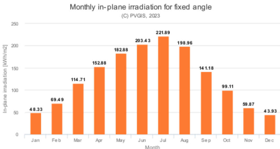
Слика 5. Просечна ирадијација при фиксен агол за дадената локација изразена во во kWh/m 2
