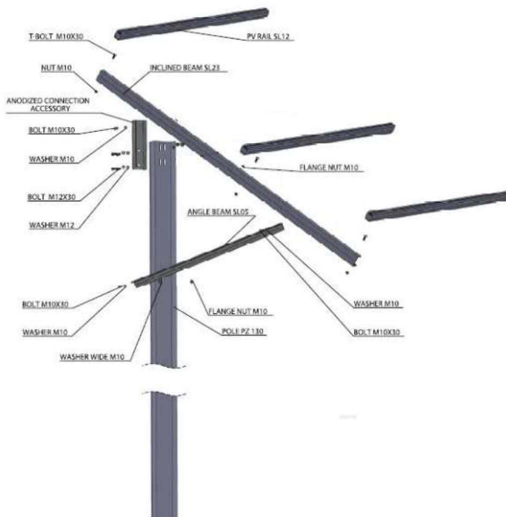
Слика 13. Приказ на целата монтажна конструкција
